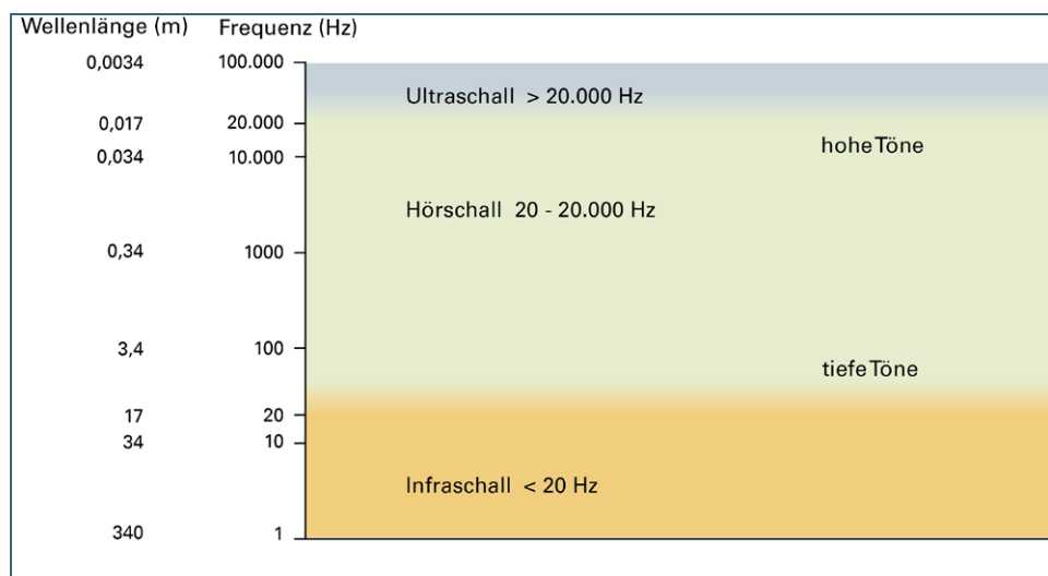
Abb. 1: Wie gut ein Mensch den ihn umgebenden Schall hört, hängt auch von dessen Frequenz ab.
