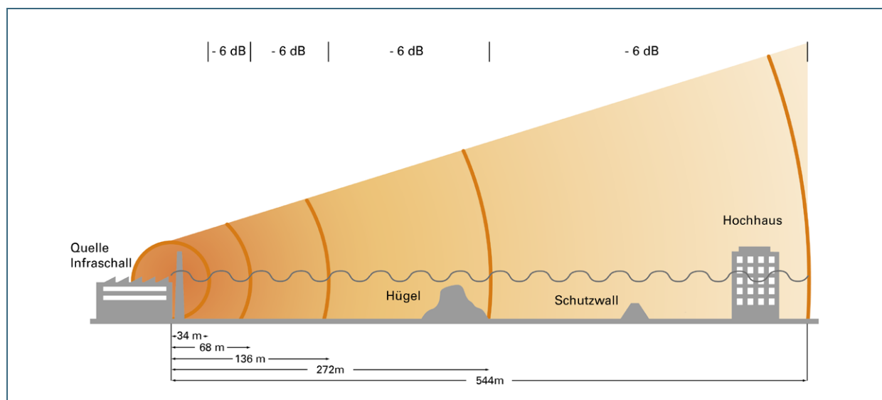
Abb. 4: Wohnhäuser, Bäume und Schutzwälle dämpfen Infraschall kaum, da seine Wellenlänge größer ist als die Hindernisse hoch sind. Der Schallpegel sinkt dann unabhängig von der Bebauung oder dem Gelände: Verdoppelt sich die Entfernung, nimmt er um sechs Dezibel (dB) ab. Im Beispiel dargestellt ist Infraschall von zehn Hertz; er hat eine Wellenlänge von 34 Metern.
